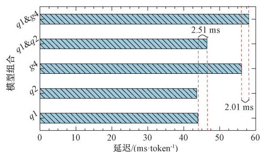
图 11 不同模型组合下的时延比较
