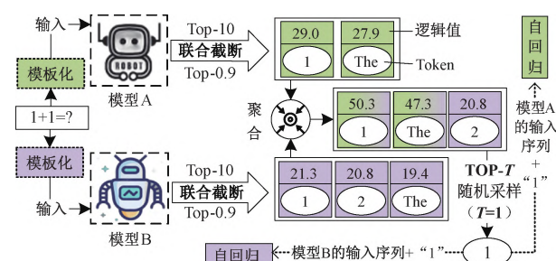
图 5 DuetNet 中模型协作推理的生成步骤示例
