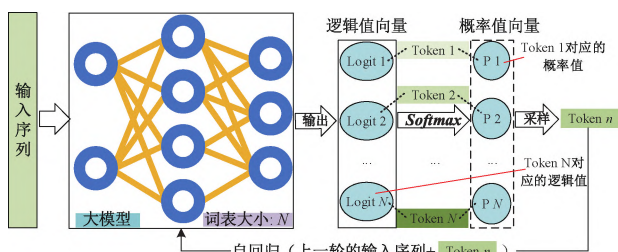
图4 大模型的自回归生成图示
